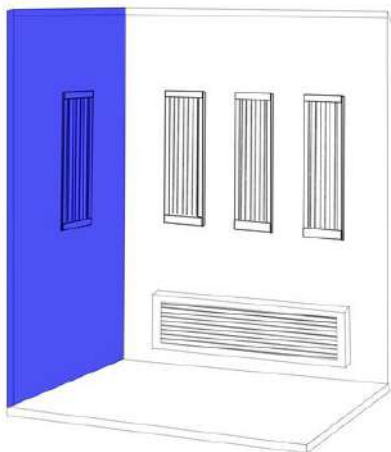
(3) Ustaw lewą ścianę na panelu podłogowym i połącz ściany klamrami
